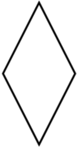
losange
