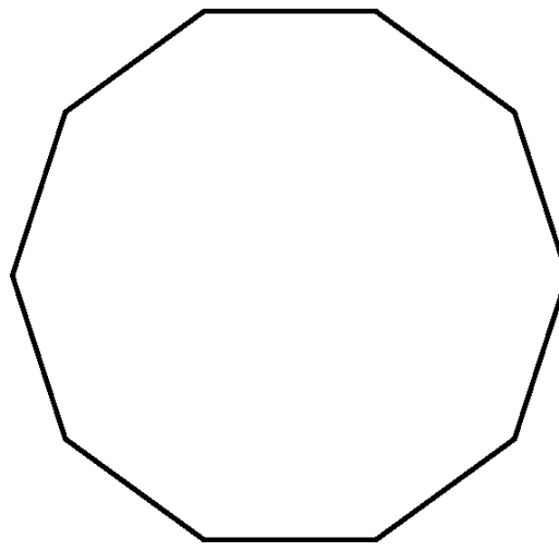
décagone
