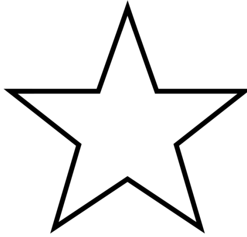
étoile
