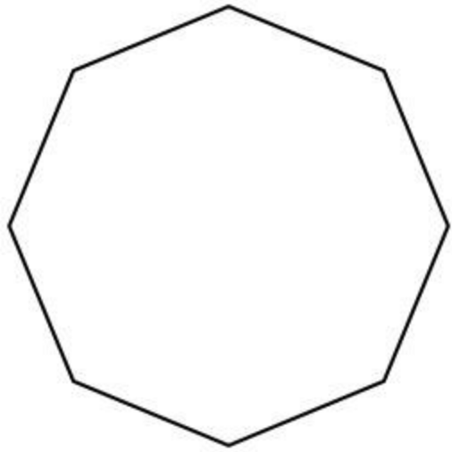
octogone
