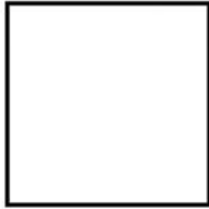
carré
