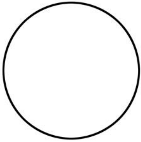
disque
