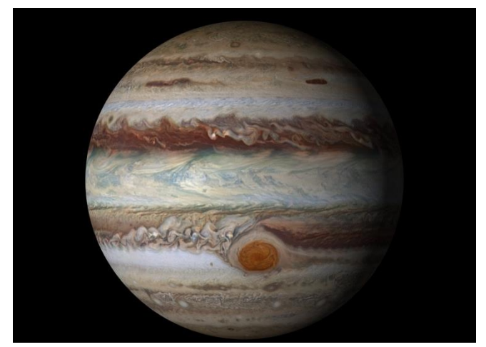
Jupiter
