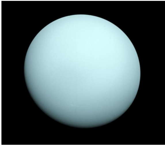
Uranus
